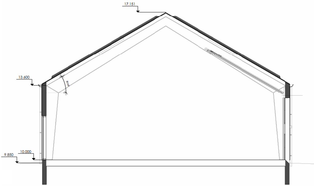
Snittegning
